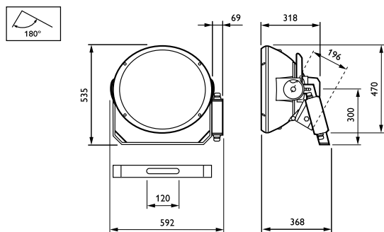
MVF404 MHN-SEH2000W/956 B5 HRE
