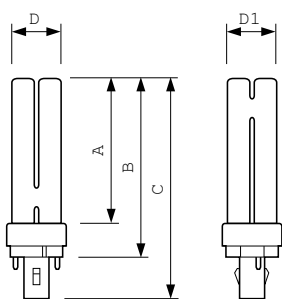
PL-C 13W/827/2P
